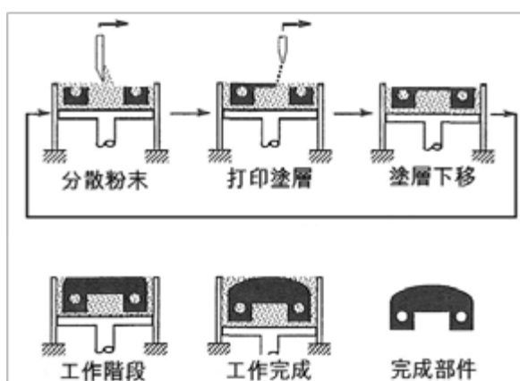
圖一：三維打印操作順序
