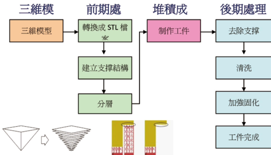
圖 1. 三維打印技術工作程序
