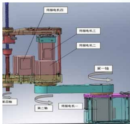
圖 8 我們研發的 SCARA 機器人
